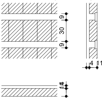
Detalhe 1 (esc. 1:30)
